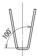
A-A 断面図
