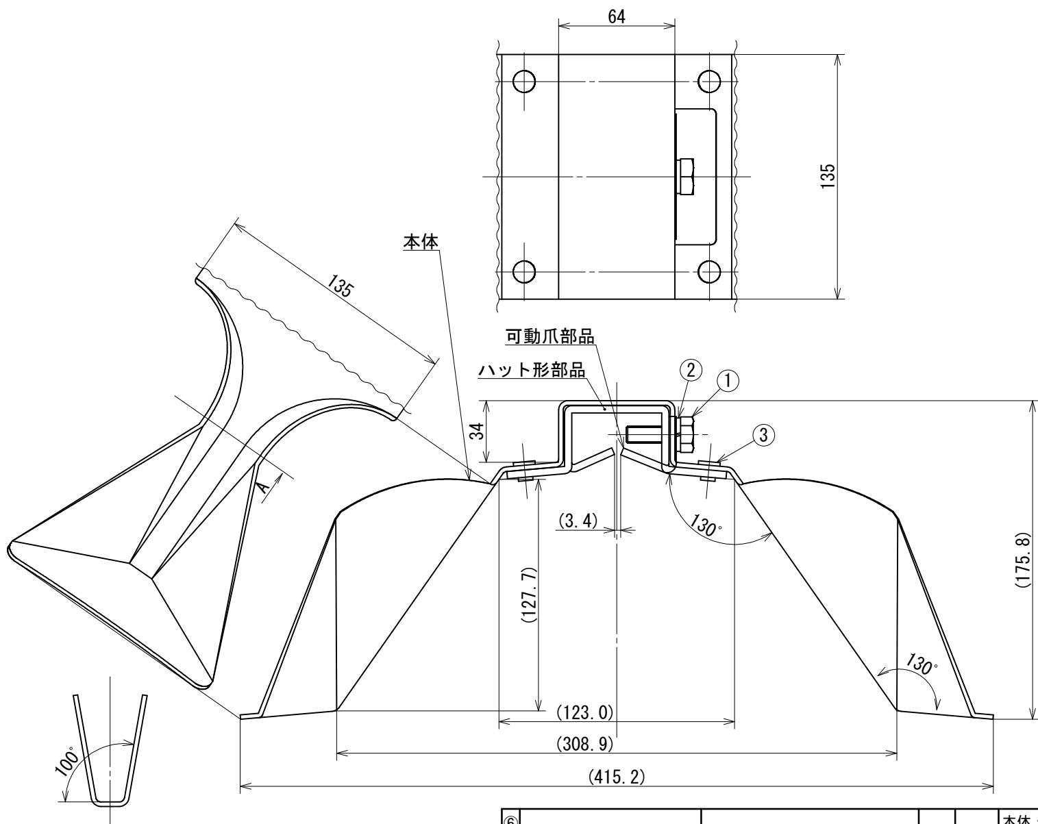
A-A 断面図
