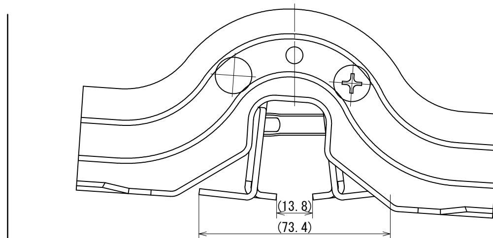
取付前形状図
