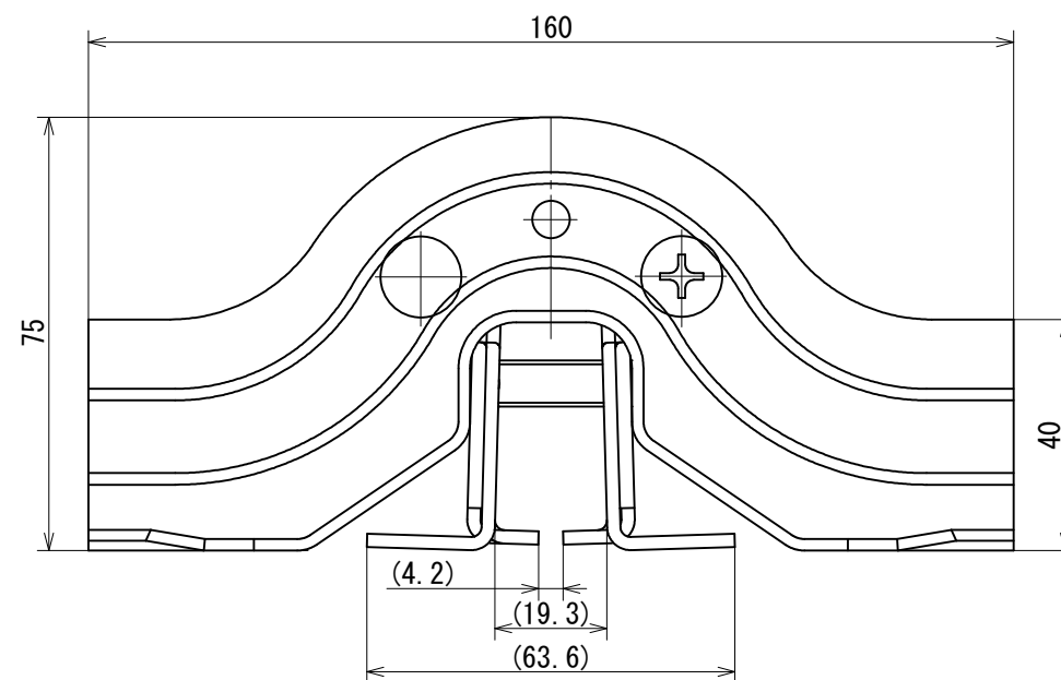
取付前形状図
