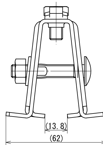
取付前形状図
