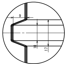
A部拡大図 スケール1/1
