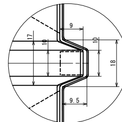
B部拡大図 スケール1/1
