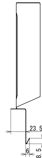
断面A-A'
