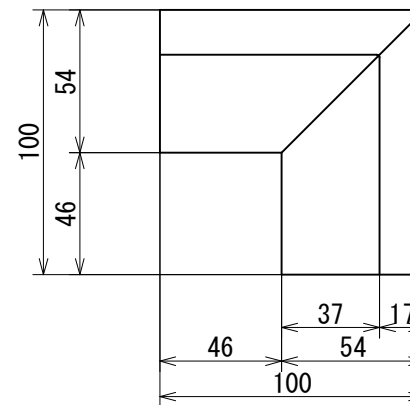
矢視B
