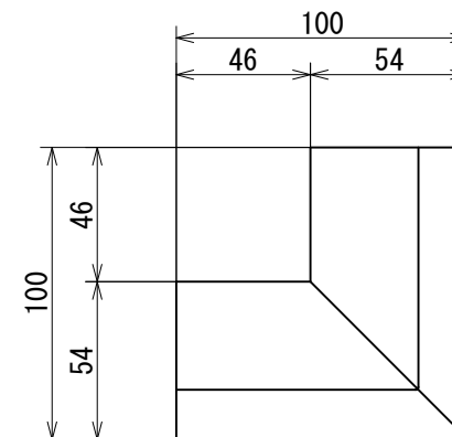
矢視A
