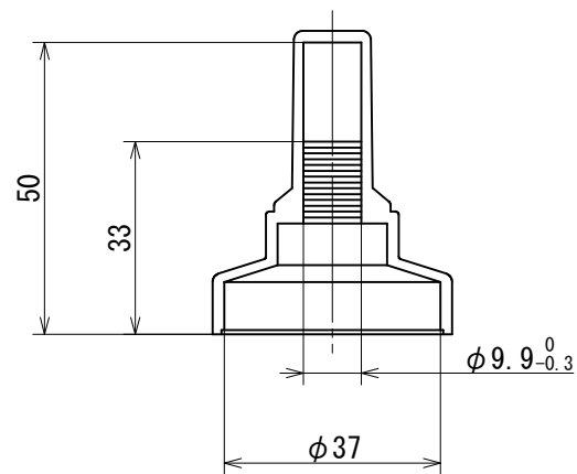
断面A-A
