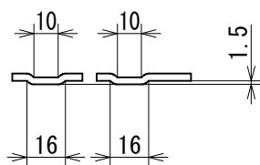
断面A-A
