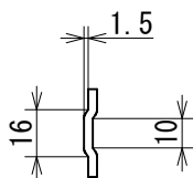
断面B-B
