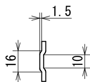
断面B-B
