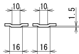
断面A-A
