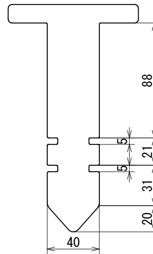
アングル押さえ金具
