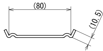
断面A-A
