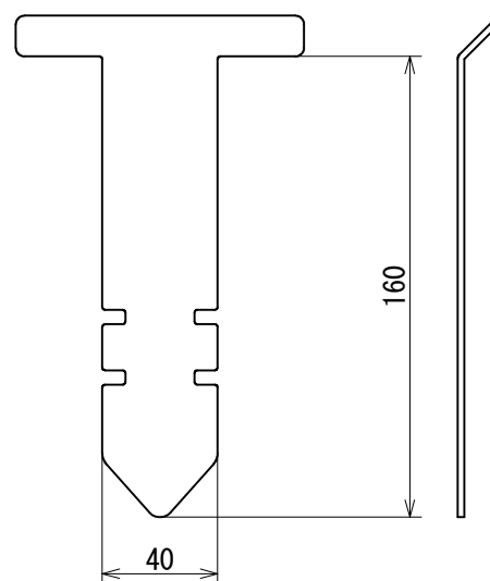
アングル押さえ金具
