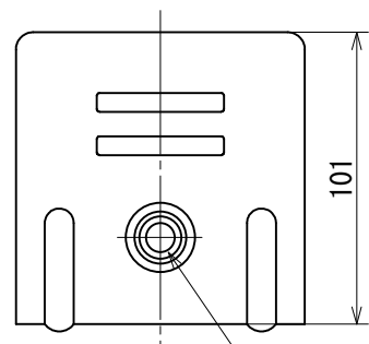
M10バーリングタップ
