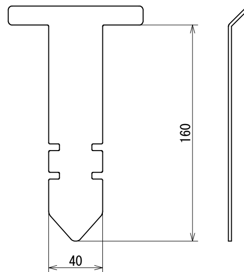
アングル押さえ金具
