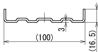
断面B-B
