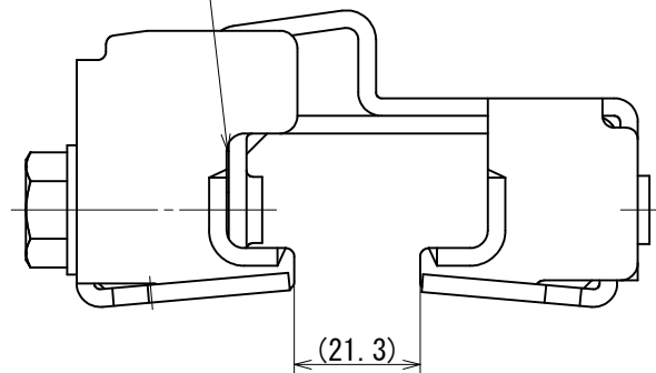
開放状態
