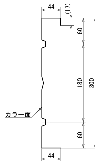
矢視 B
