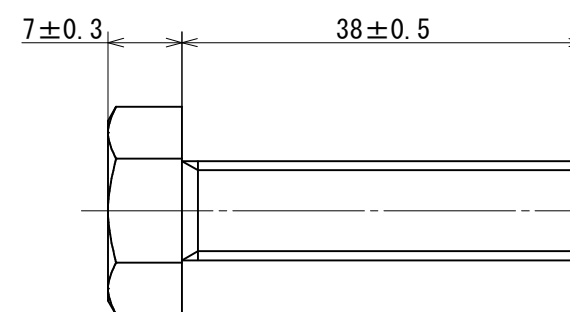
六角ボルト
