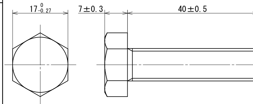
六角ボルト
