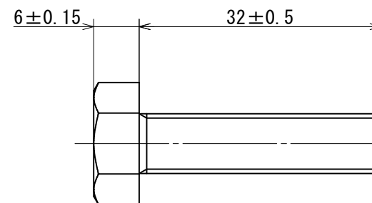
六角ボルト
