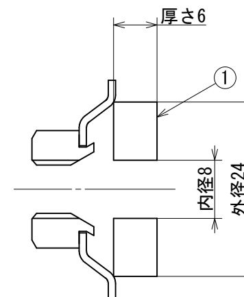
断面A-A
