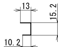
断面C-C
