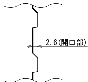
断面A-A
