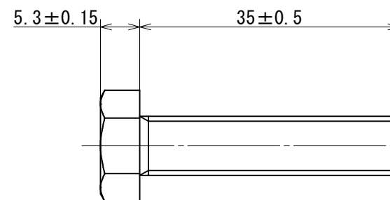
六角ボルト
