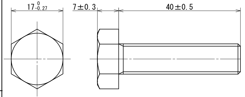
六角ボルト
