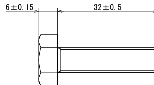
六角ボルト
